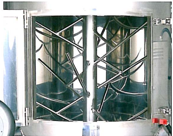
▲ 枝式スクリュー
